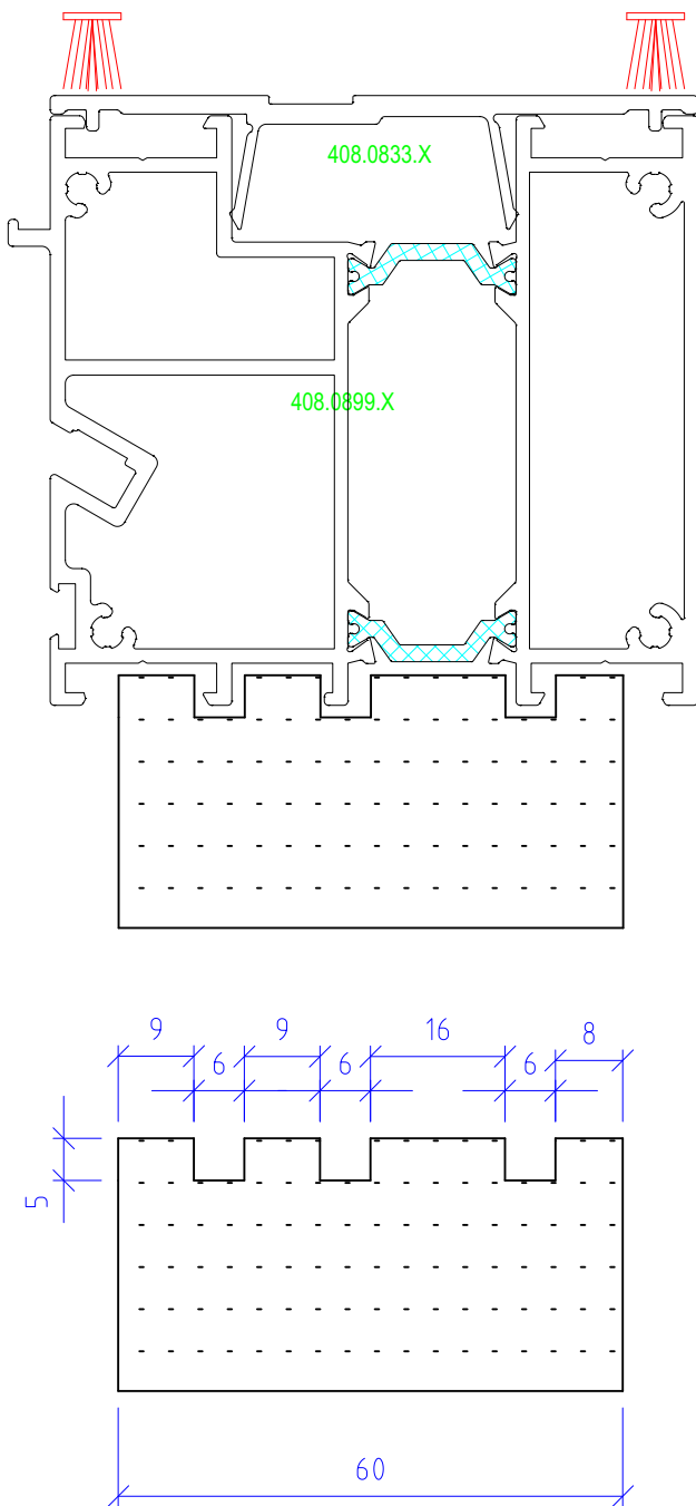
PURBASE-Drzwi Pivot Masterline 8 wymiary w [mm]
